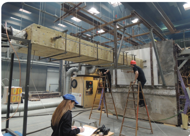
Obr. 16 Měření deformace potrubí typu C při zkoušce ve zkušebně
