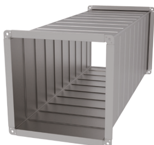
Obr. 64 Maximální rozměr potrubí, které se nevyztužuje, je 500 × 500 mm, délka segmentu 1500 mm
