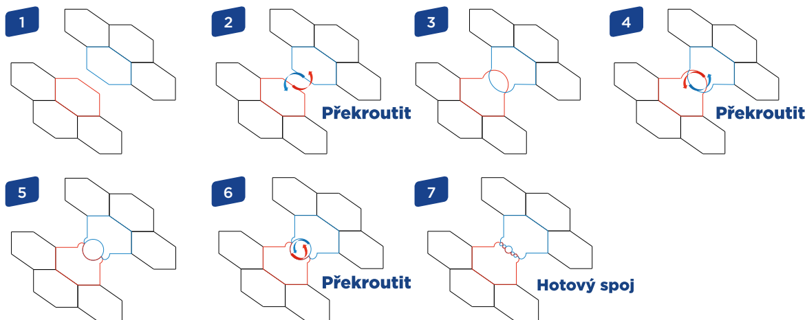
Obr. 62 Schematické znázornění principu spojení rohože na pleťivu
