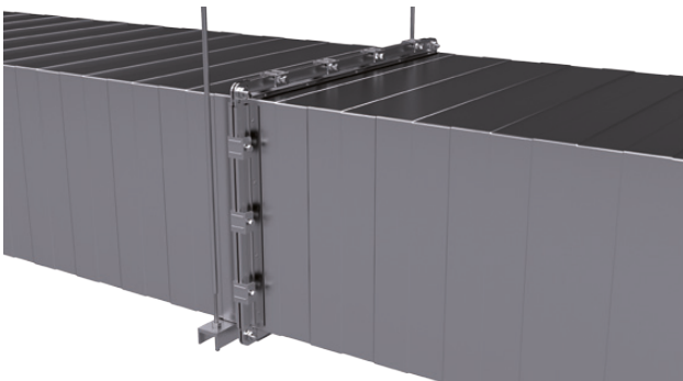
Obr. 41 Závěsné zařízení možno s výhodou umísťovat do těsné blízkosti přírub
