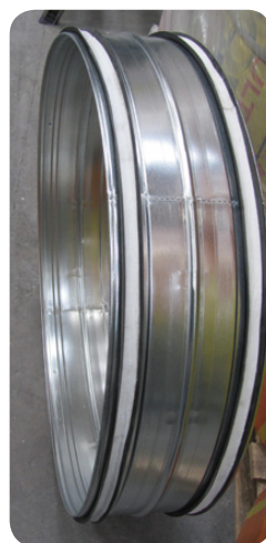
Obr. 57 Keramická páska 20 × 3 mm vložena mezi EPDM těsnění
