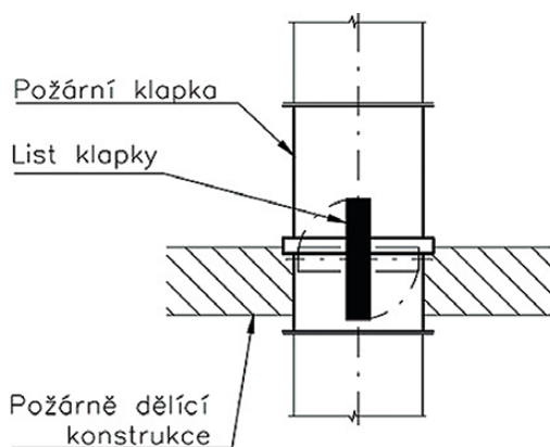
Obr. 84 Požární klapka zabudovaná přímo v požárně dělicí konstrukci svislé nebo vodorovně
