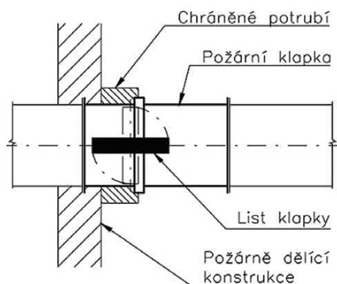
Obr. 85 Požární klapka zabudovaná mimo požárně dělicí konstrukci; část potrubí od požárně dělicí konstrukce po list klapky musí být chráněna protipožární izolací dle pokynů výrobce požární klapky dané výsledkem zkoušky ČSN EN 1366-2, nelze montovat izolaci testovanou dle ČSN EN 1366-1!
