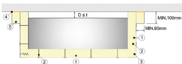
Obr. 80 Příčný řez vodorovným potrubím s izolací na 3 stranách
