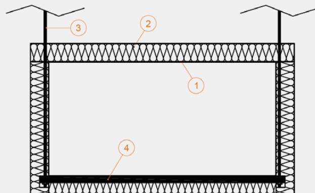
Obr. 22 Závitové tyče uvnitř izolace
