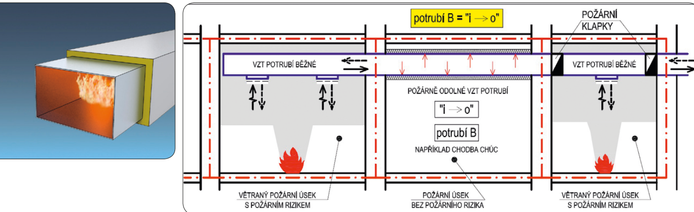
Obr. 7 Příkladem, kdy se požaduje provedení vzduchotechnického potrubí namáhaného požárem z vnitřní strany (potrubí B), je také zařízení, které větrá prostor s požárním rizikem (např. sklady) a vzduchovod dále prochází bez vyústek chráněnou únikovou cestou. Úsek vzduchovodu v CHŮC pak musí být odolný působení požáru z vnitřní strany.
