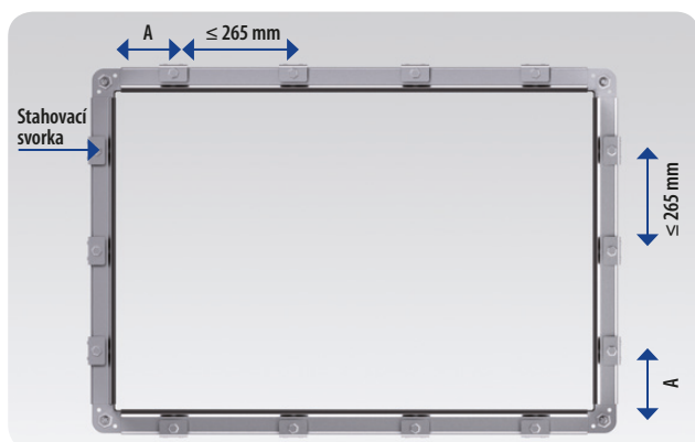
Obr. 69 Rozmístění stahovacích svorek
