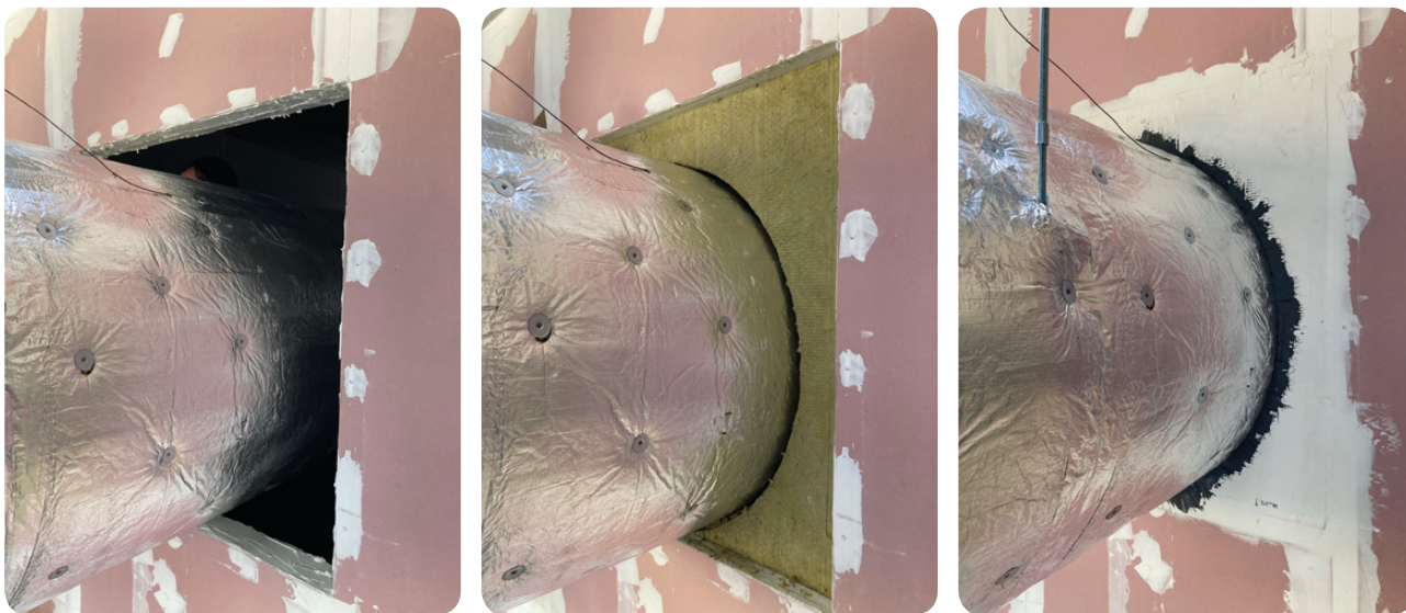
Obr. 35 Provedení měkké požární ucpávky
