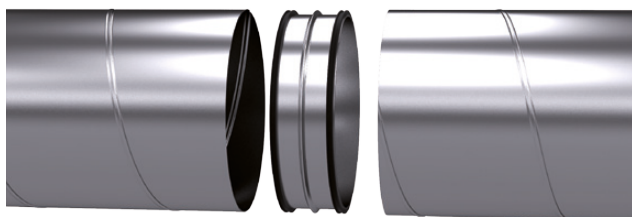
Obr. 56 Vsuvka Lindab Safe s oboustranným lemováním EPDM těsněním
