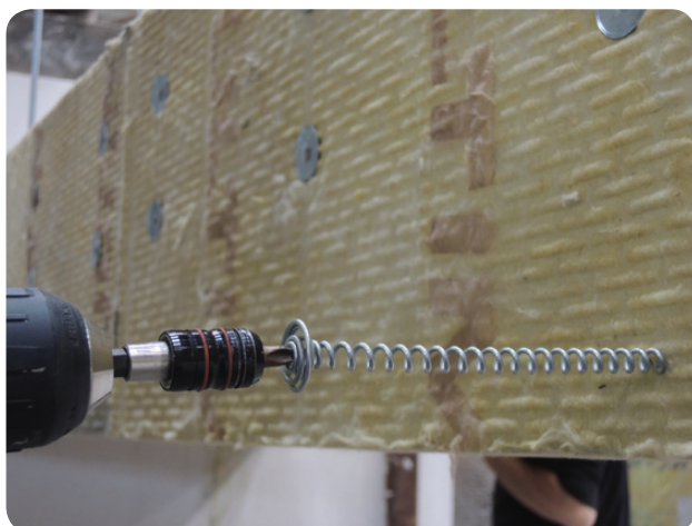
Obr. 73 Rohové styky desek jsou spojeny požárními vruty Fire Screw
