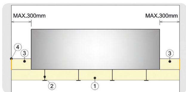
Obr. 77 Příčný řez svislým potrubím s izolací z 1 strany
