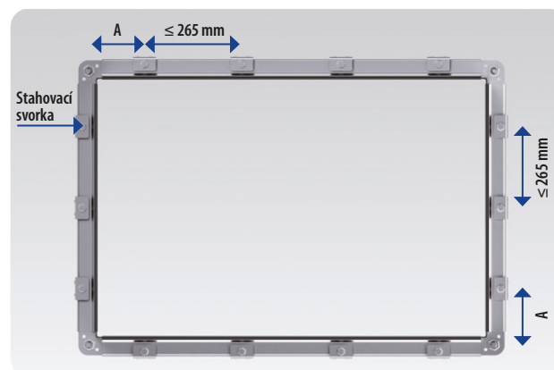
Obr. 40 Příruby zajištěné stahovacími svorkami
