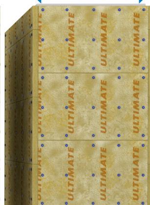
Obr. 45 Rozmístění trnů a vrutů u svislého potrubí
