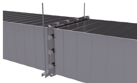
Obr. 70 Závěsné zařízení je možno s výhodou umířovat do těsné blízkosti přírub
