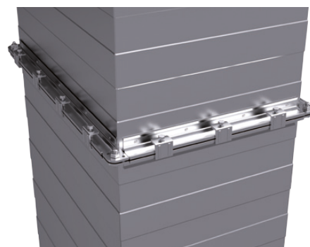
Obr. 39 Příruby zajištěny stahovacími svorkami
