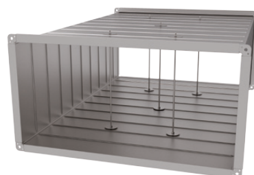
Obr. 65 Stanovení počtu výztuh pro potrubí 1000 × 500 mm, délka segmentu 1500 mm: (1 × 1,5) m 2 : 0,3 m 2 /výztuhu = 5 výztuh rovnoměrně rozmístěných v ploše
