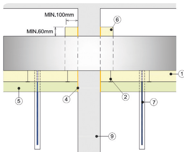
Obr. 82 Podélný řez potrubím s izolací na 2 stranách procházející požárně dělicí konstrukcí
