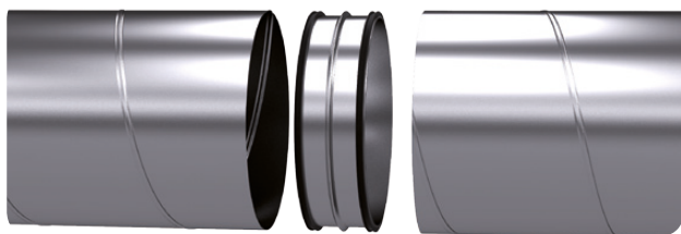
Obr. 63 Vsuvka Lindab Safe s oboustranným lemováním EPDM těsněním, obě strany potrubí musí být pro případ požáru utěsněny keramickou páskou
