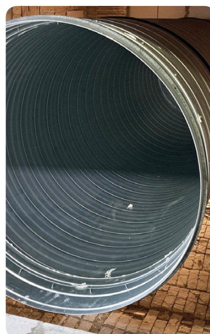
Obr. 33 Pohled na spiro potrubí spojované vsuvkami, oba konce vsuvky jsou opatřeny intumescentním akrylátovým tmelem
