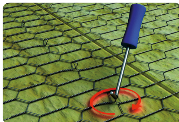
Obr. 61 Spojení rohoží překroucením přiléhajících okrajů pleťiva do sebe po vzdálenosti cca 100 mm
