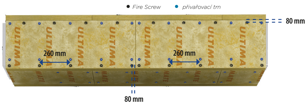
Obr. 72 Maximální vzdálenosti trnů a vrutů Fire Screw
