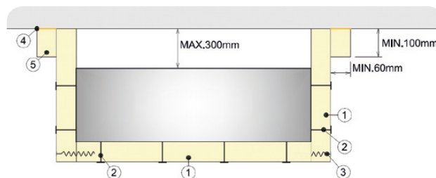
Obr. 51 Příčný řez svislým vzduchodem s izolací na 3 stranách
