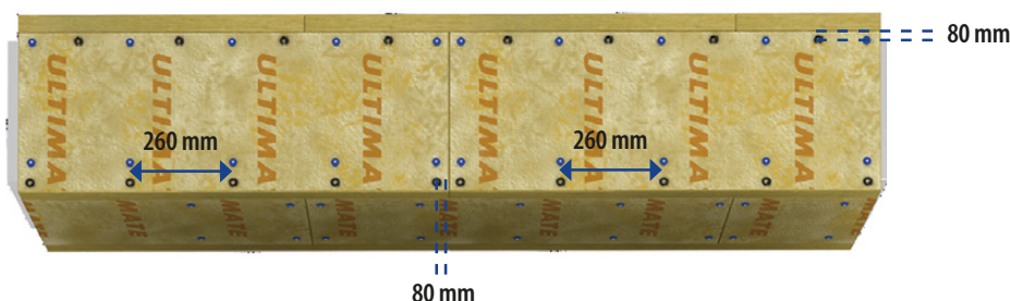
Obr. 43 Maximální vzdálenosti trnů a vrtů Fire Screw
