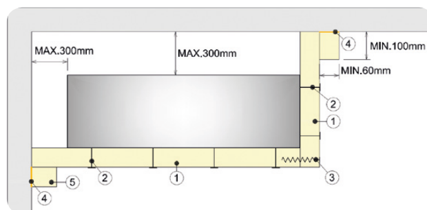
Obr. 50 Příčný řez vzduchodem s izolací na 2 stranách
